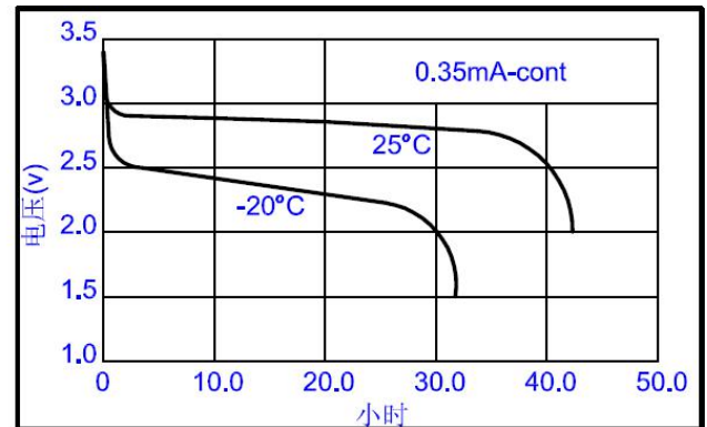
恒流放电曲线
