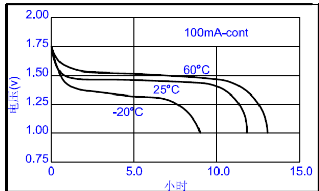
恒流放电曲线
